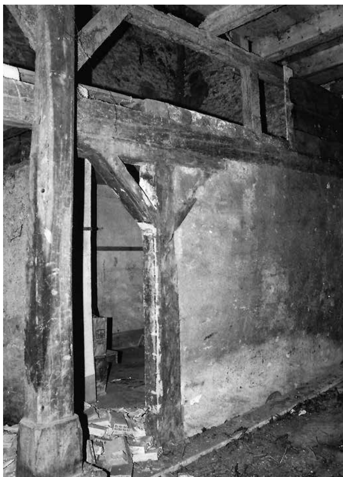
18 Der Mittelposten im Kernbau ist datiert. Er unterstützte ursprünglich die Firstpfette oder ein Podest, das das Befüllen der Mostpresse erleichterte. Foto, 1984 (FLM 104.02).
