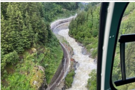
Unterspülung MGBahn-Streckennetz bei St. Niklaus
