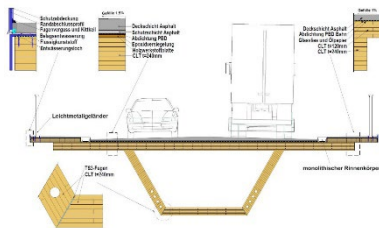
Bild 2: Möglicher Aufbau und Details eines Brückenquerschnitts mit mittlerer Spannweite (Arbeitsmodell)
